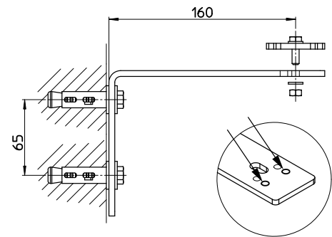
DN32 - 160 mm
