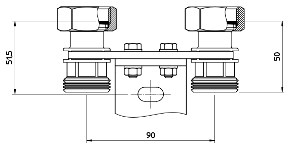
DN20
