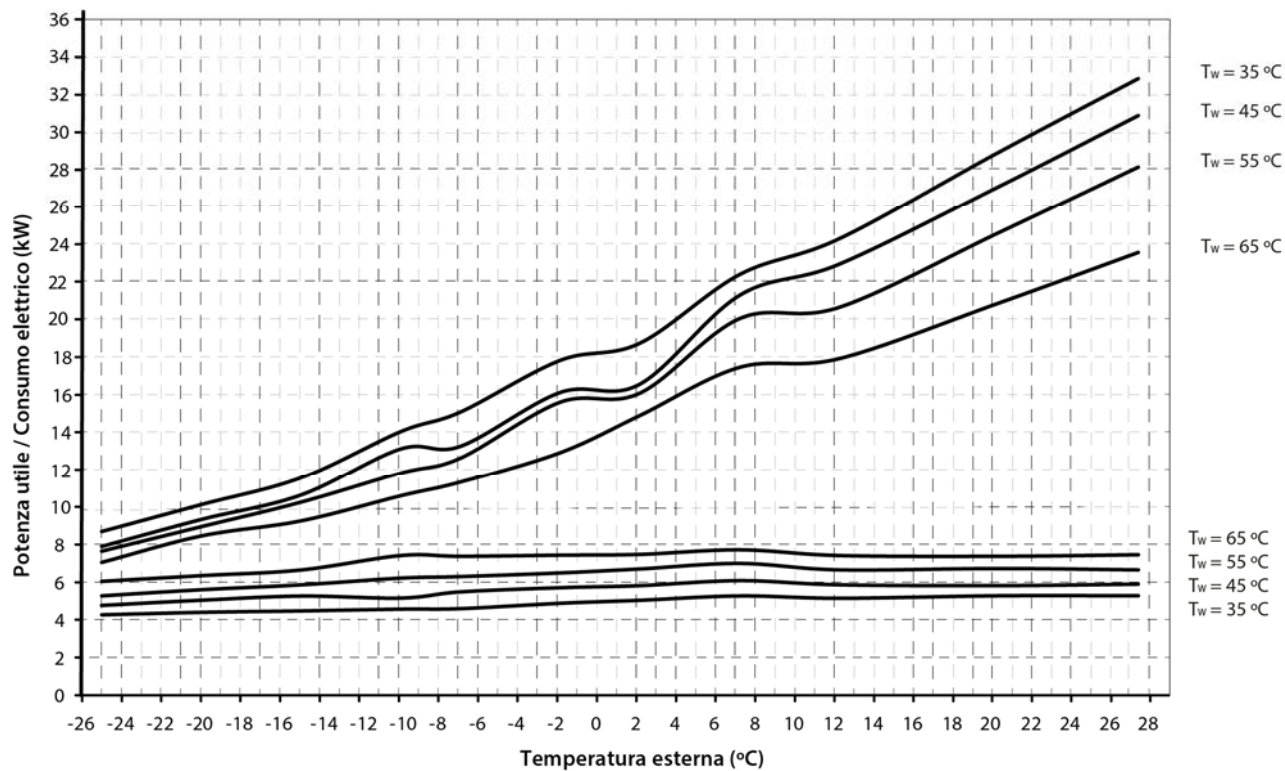
Curve di prestazioni in riscaldamento Dual Clima 22HTT
