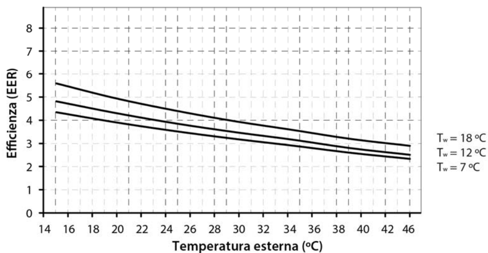
Curve di efficienza in raffreddamento Dual Clima 19HT/19HTT (EER)
