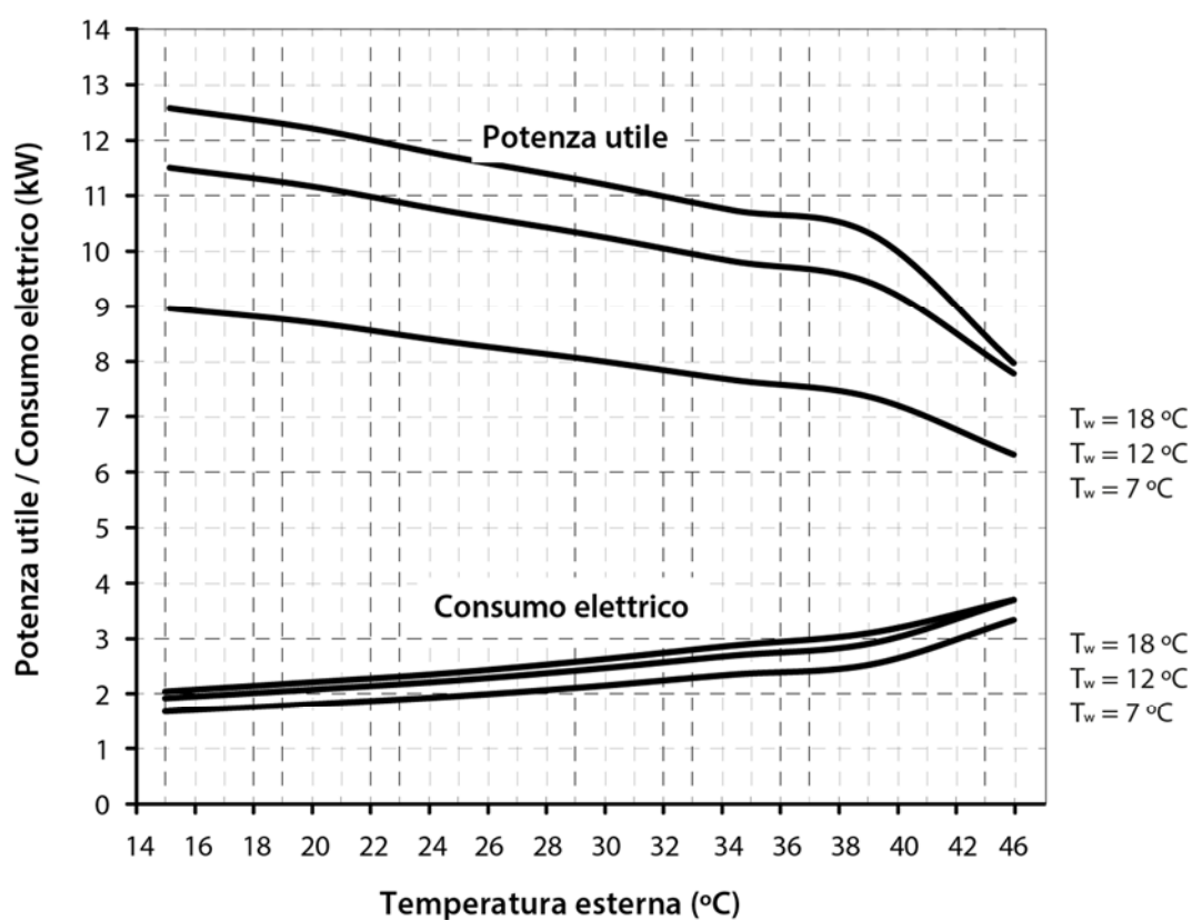
Curve di prestazioni in raffreddamento Dual Clima 12HT/12HTT
