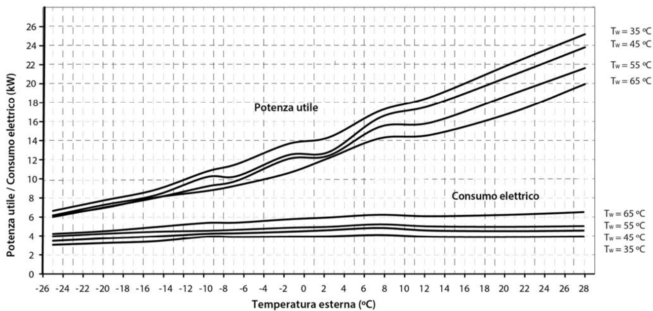
Curve di prestazioni in riscaldamento Dual Clima 16HT/16HTT
