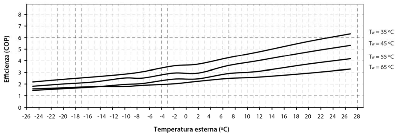
Curve di efficienza in riscaldamento Dual Clima 16HT/16HTT (COP)
