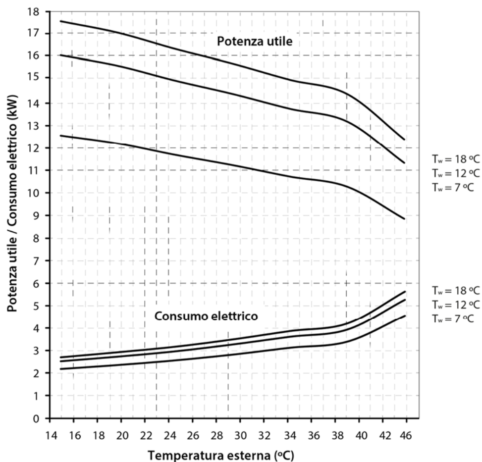
Curve di prestazioni in raffreddamento Dual Clima 16HT/16HTT
