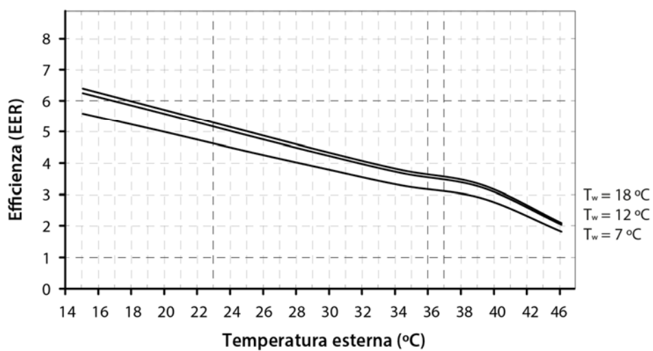
Curve di efficienza in raffreddamento Dual Clima 16HT/16HTT (EER)
