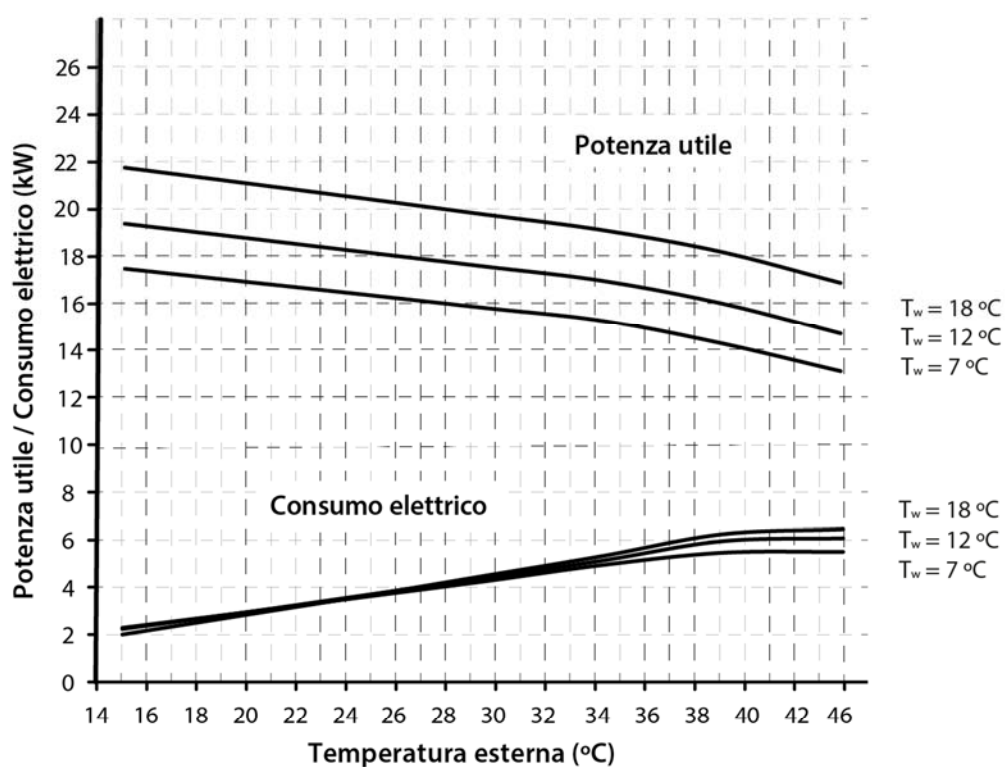
Curve di prestazioni in raffreddamento Dual Clima 19HT/19HTT
