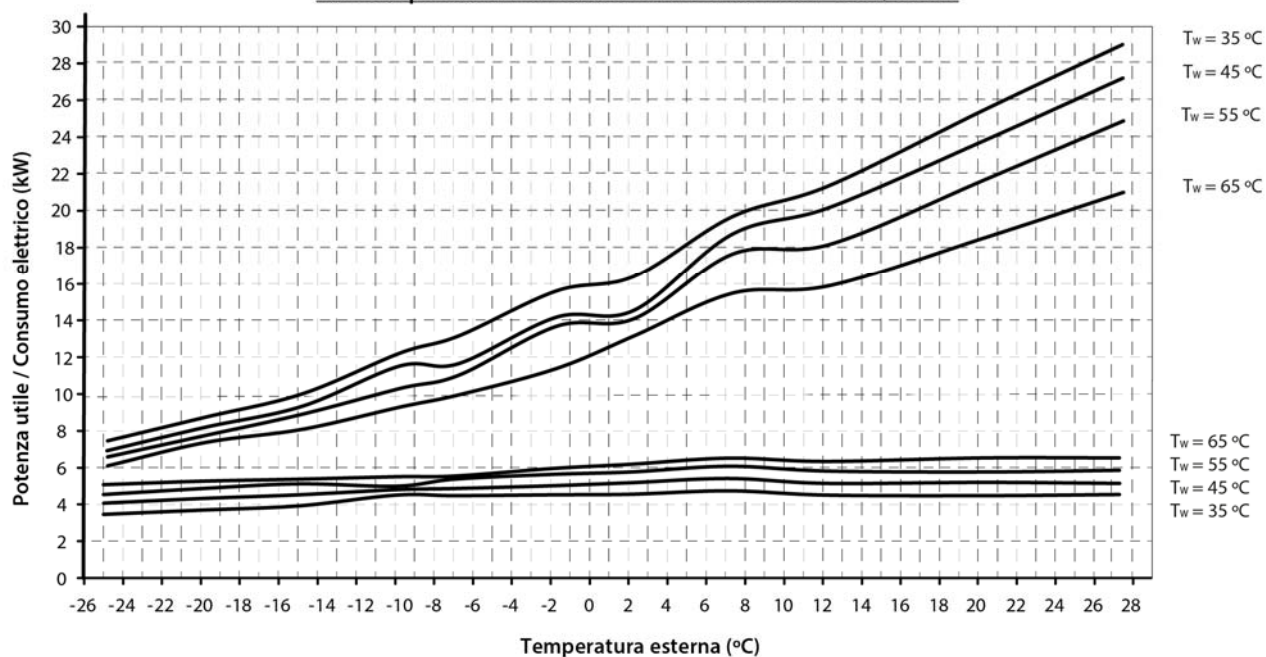
Curve di prestazioni in riscaldamento Dual Clima 19HT/19HTT
