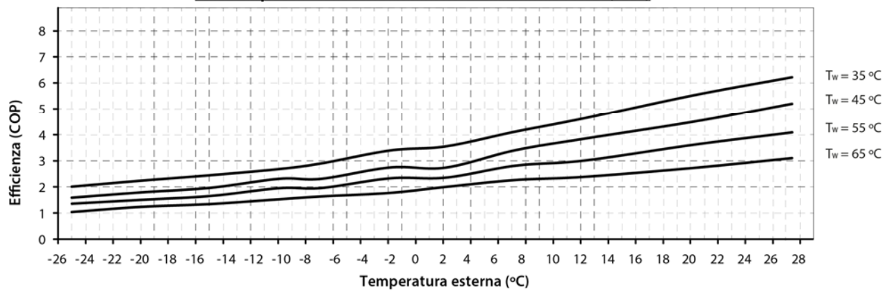
Curve di prestazioni in riscaldamento Dual Clima 22HTT (COP)
