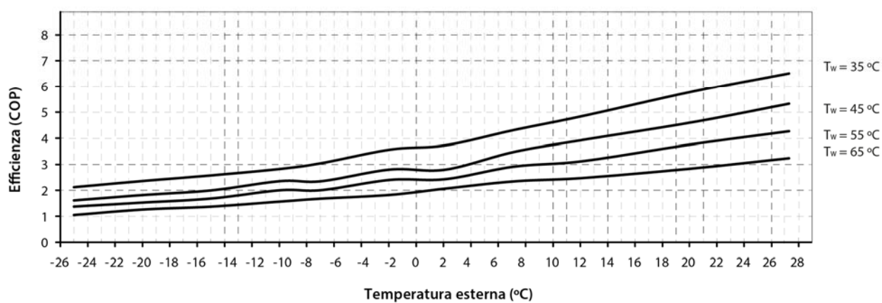
Curve di prestazioni in riscaldamento Dual Clima 19HT/19HTT (COP)
