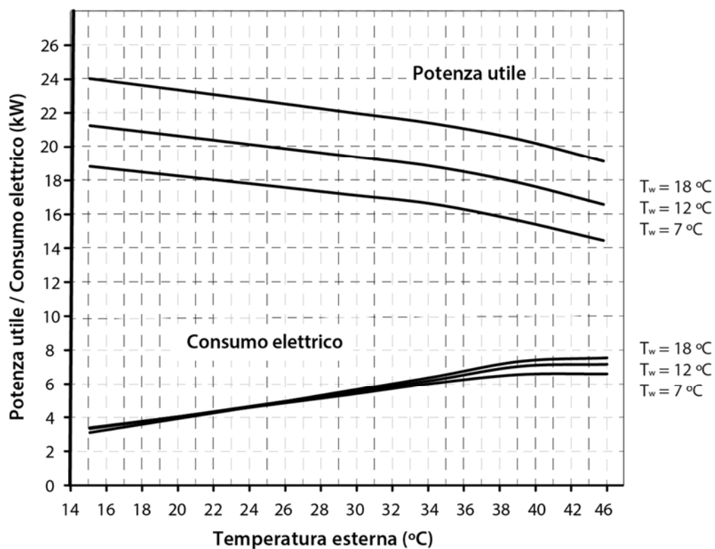
Curve di prestazioni in raffreddamento Dual Clima 22HTT
