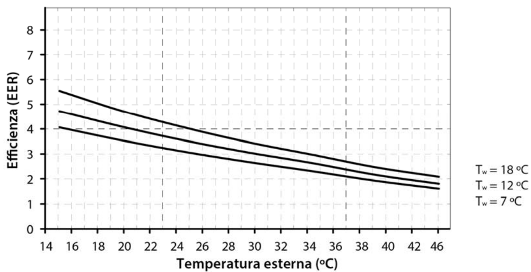
Curve di efficienza in raffreddamento Dual Clima 22HTT (EER)
