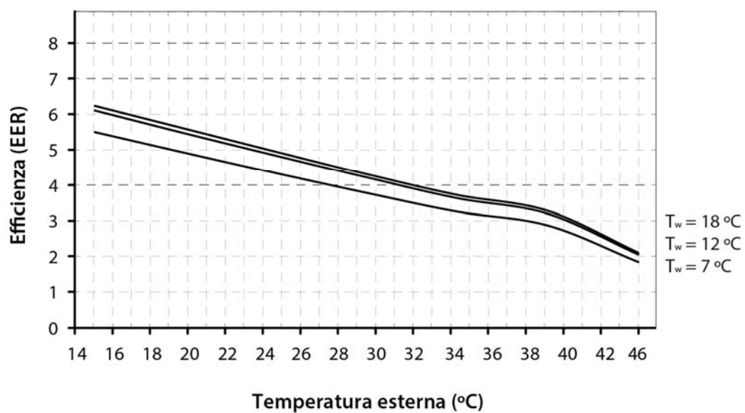
Curve di efficienza in raffreddamento Dual Clima 12HT/12HTT (EER)
