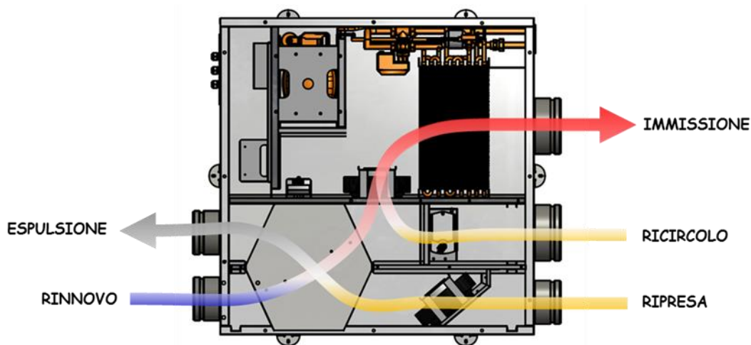
Figura 2 - Schema flussi unità (vista lato ispezione, quindi dal basso)
