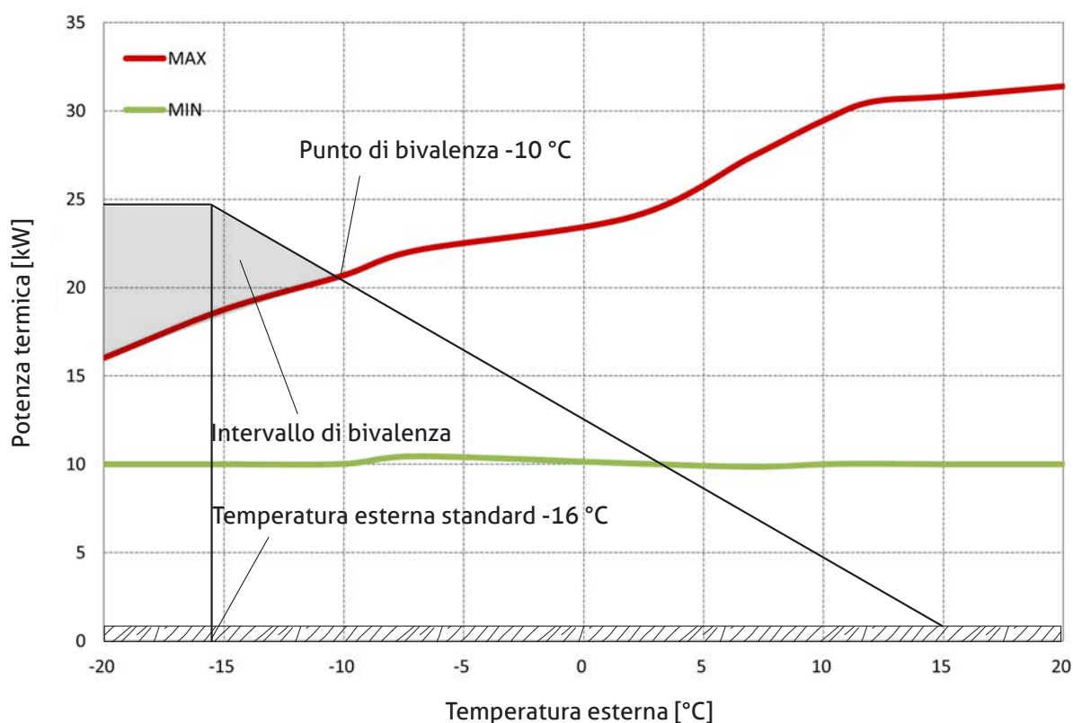
Potenza termica - Mandata 35^{\circ}\text{C}
